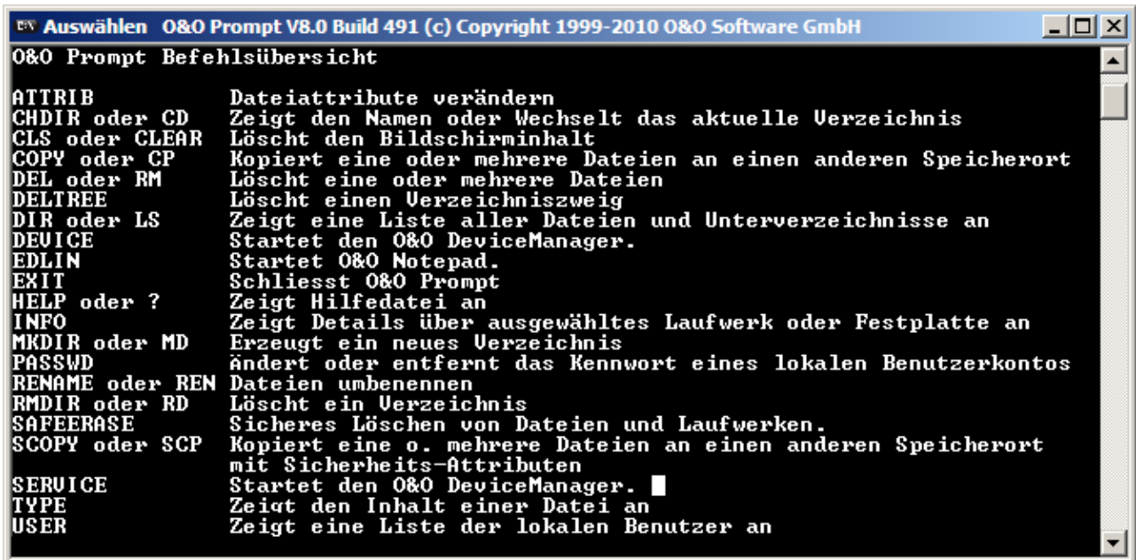
O&O Prompt: Kommandozeile
